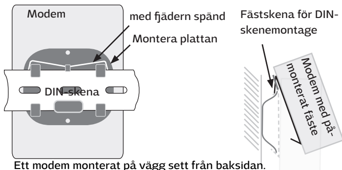
Ett modem monterat på vägg sett från baksidan.
